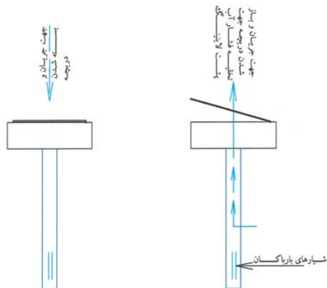
زمانیکه کانال در حال تخلیه است جهت جریان آب و بسته شدن بارباکان زمانیکه کانال در حال آنگسیری است
