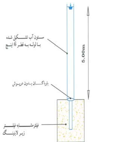
مدل فیزیکی بارباکان مورد آزمایش بدون درپوش و اندازه گیری میزان نشتی
